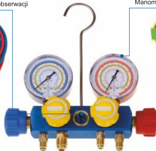
Manometr klasy 1.6
